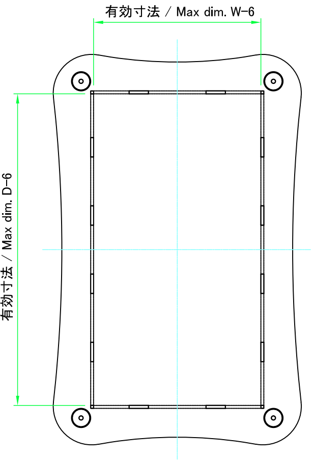
下カバー / Bottom cover
