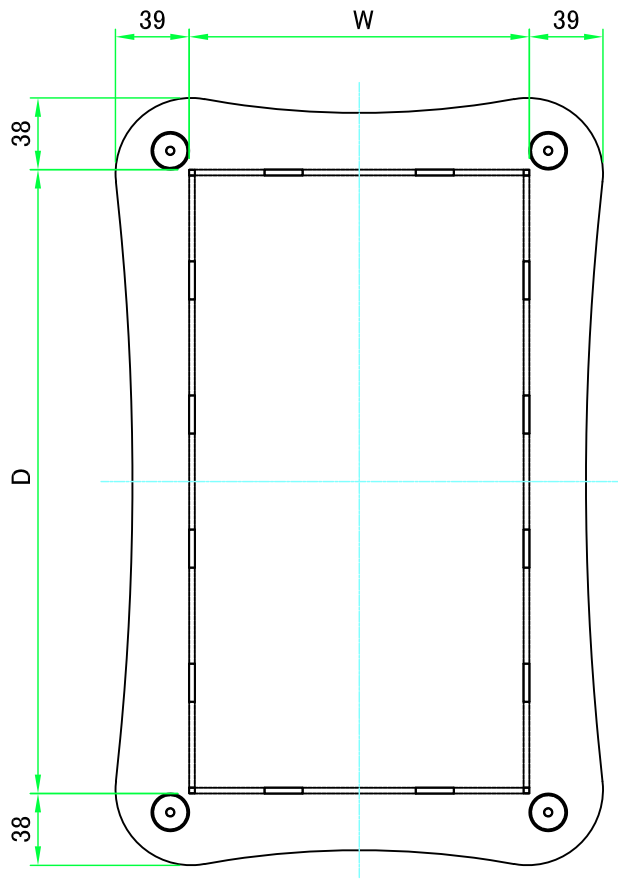
Wパネル1 / W panel 1
